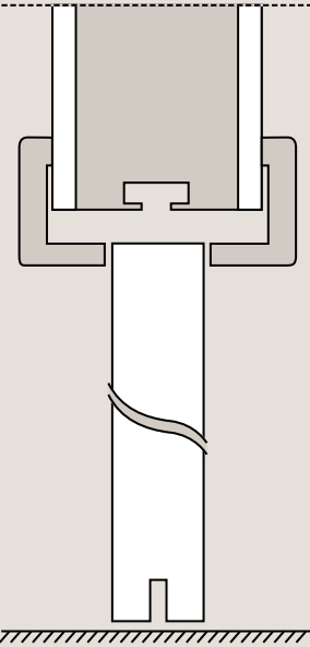
Coupe verticale
