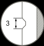
Matriçage/fraisage pour Etna en gris lave (en millimètres)
