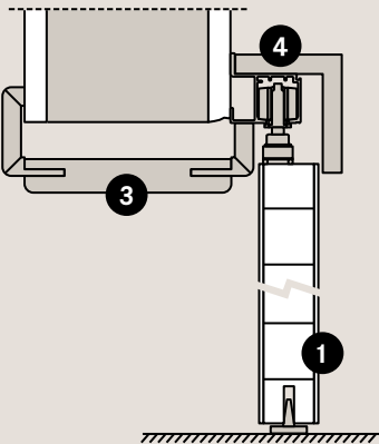
Coupe verticale
